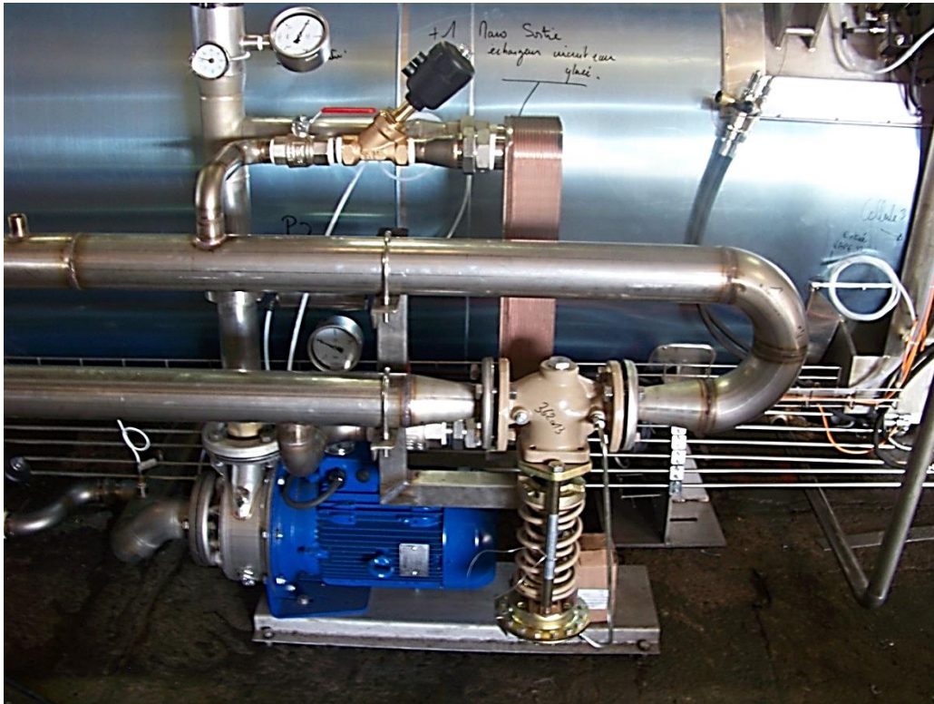
ENSEMBLE ECHANGEUR AVEC BOUCLE EAU GLACEE
