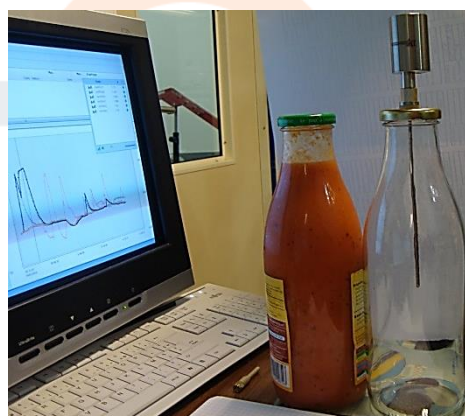
Contrôle à cœur par capteur embarqué radio
