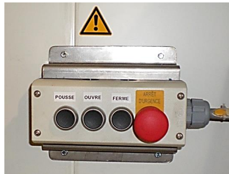
Système de commande déporté : Entrée / Sortie / Ouverture des portes Avanement des chariots
