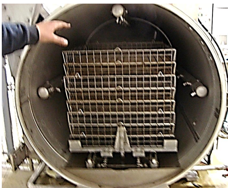
Contrôle à cœur par capteur embarqué radio
